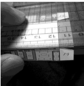
写真 3 床下機器の折り曲げ。定規で正確に。
