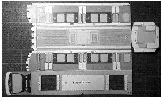
写真 5 くり抜き済の車体(表面)
