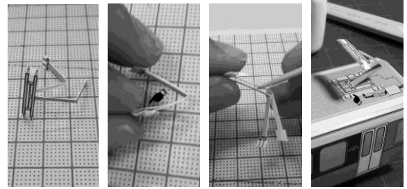
写真 20, 21, 22, 23 Z型パンタの組み立て
